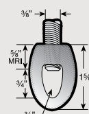
Eye Nut
