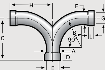
Standard Double 90° Y
